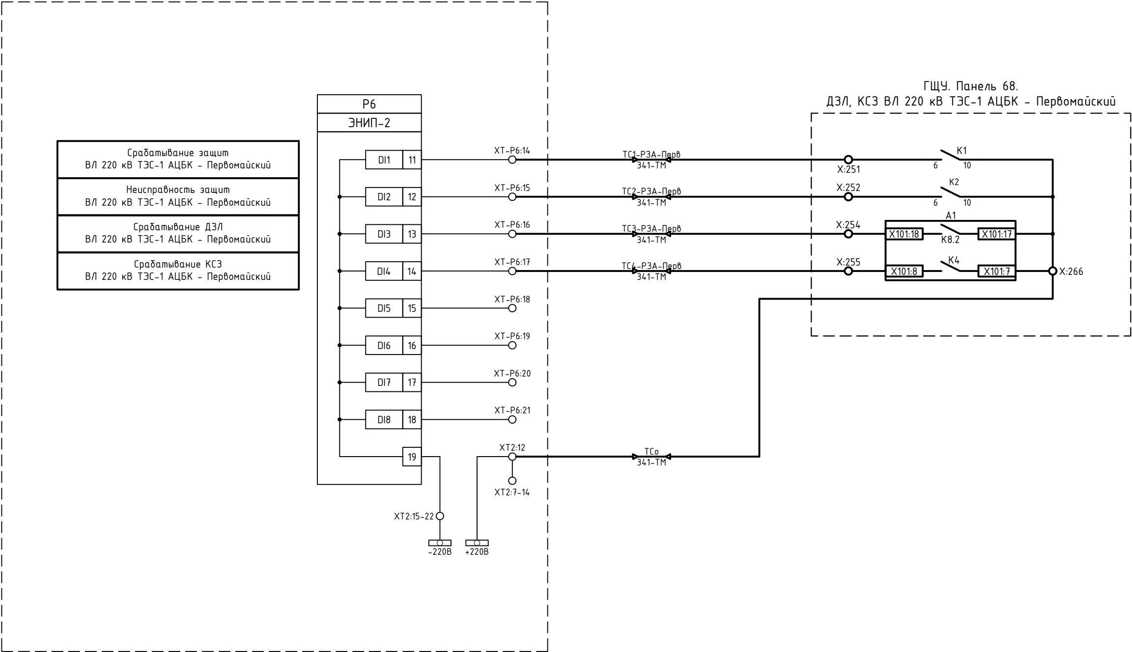
ГЩУ. Панель 71. Шкаф ССПИ-1
